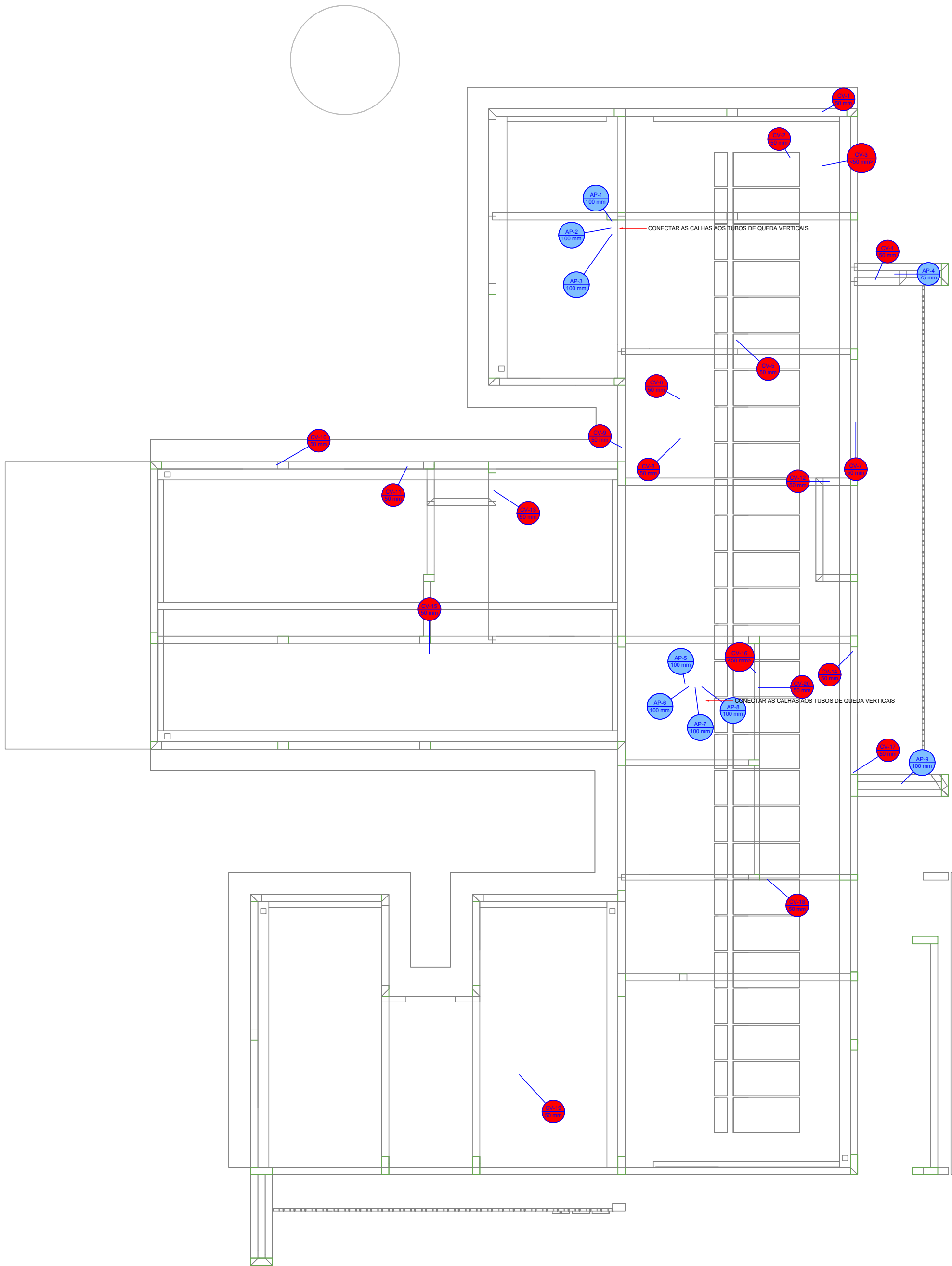
PLANTA - SANITÁRIO - COBERTURA ESC. 1/50
