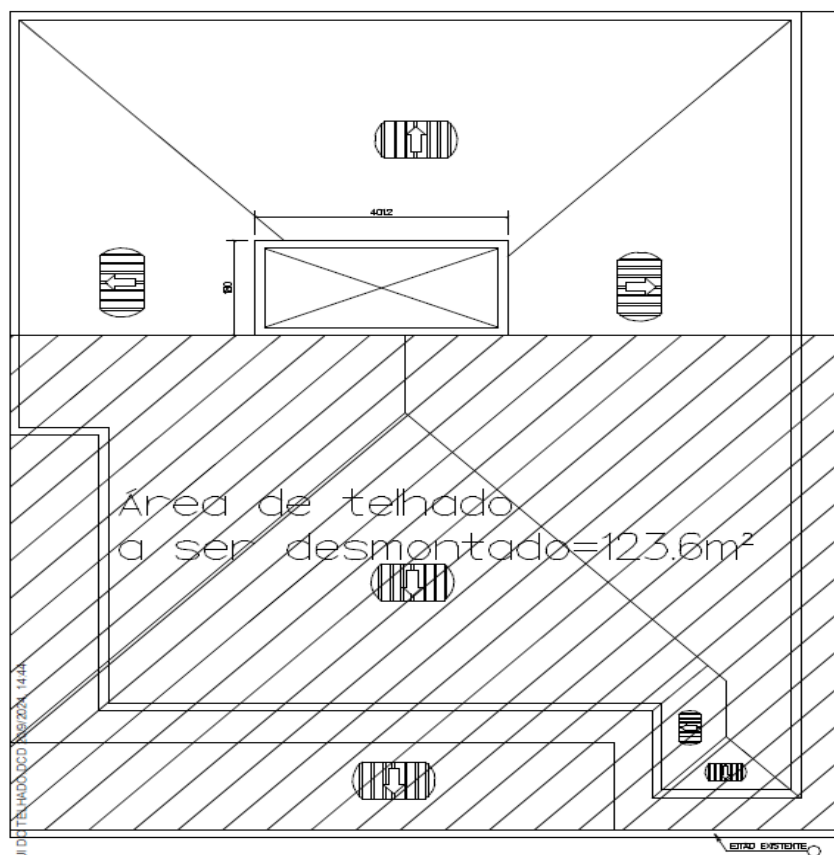
TELHADO EXISTENTE
