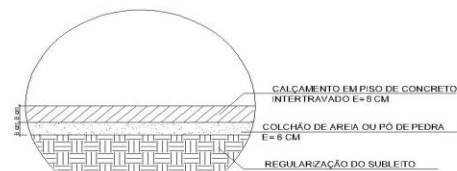
DETALHE - CAMADAS DE CALÇAMENTO Esc: Sem Escala
