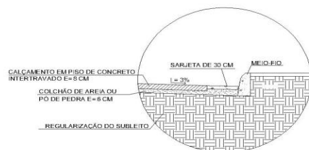
DETALHE - MEIO-FIO E SARJETA Esc: Sem Escala
