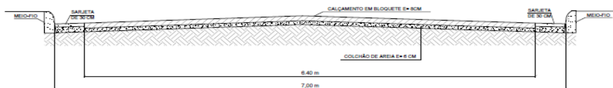
CORTE TRANSVERSAL Esc. 1:50
