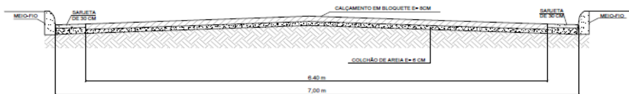
CORTE TRANSVERSAL Escala: 1:20
