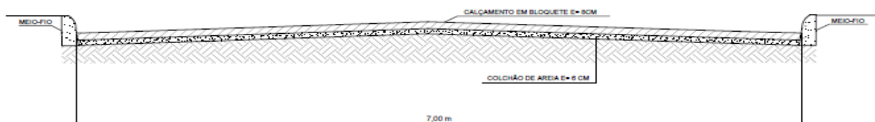
CORTE TRANSVERSAL
