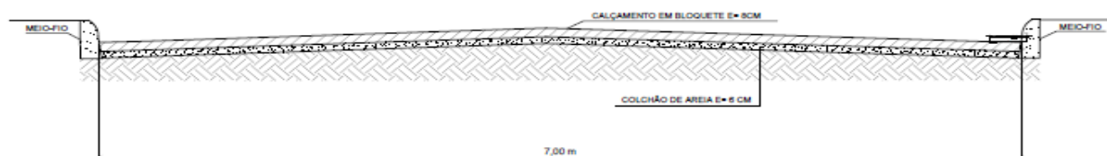
CORTE TRANSVERSAL
