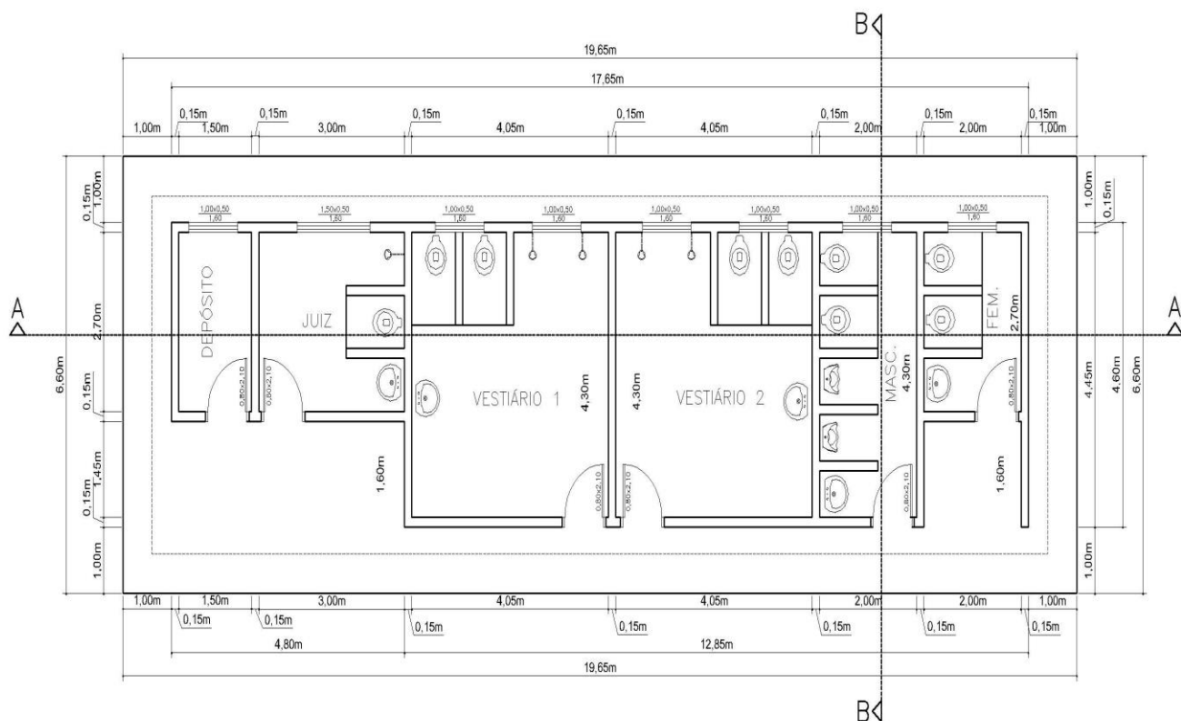
PLANTA BAIXA
