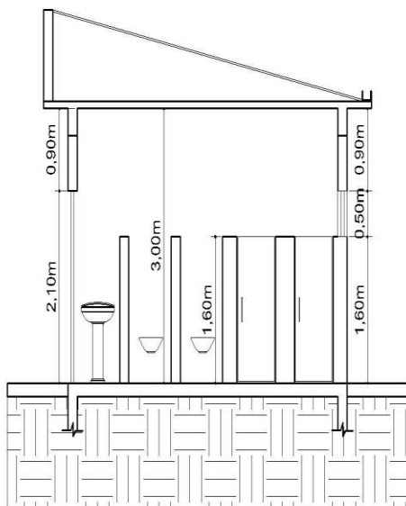
CORTE BB
